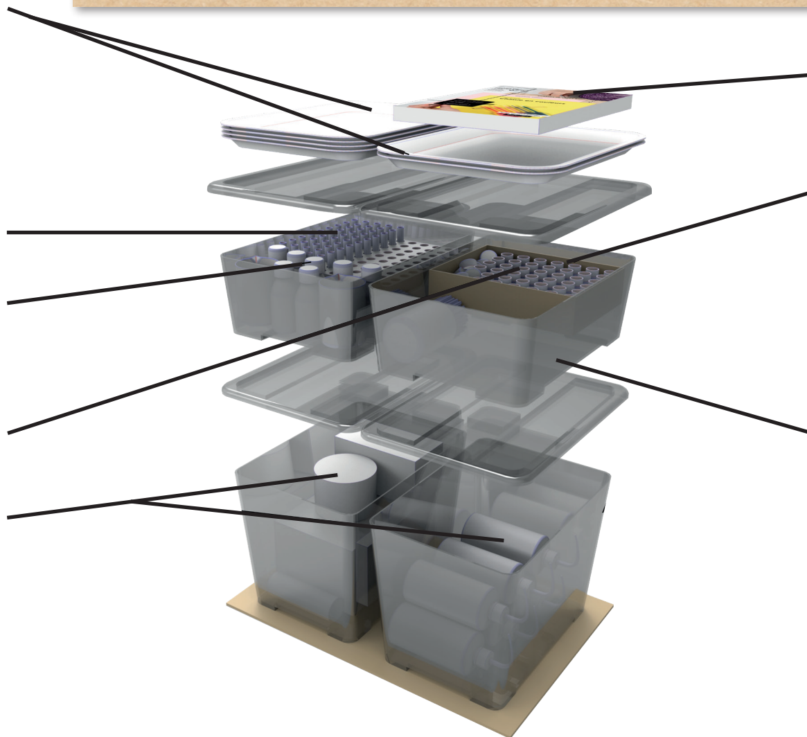
Vue en éclaté de l'intérieur de la mallette
