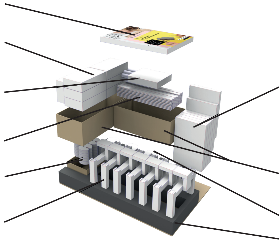
Vue en éclaté de l'intérieur de la mallette
