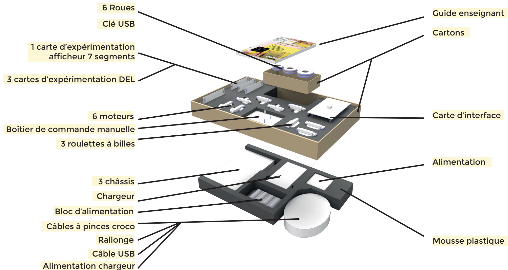
Vue en éclaté de l'intérieur de la mallette
